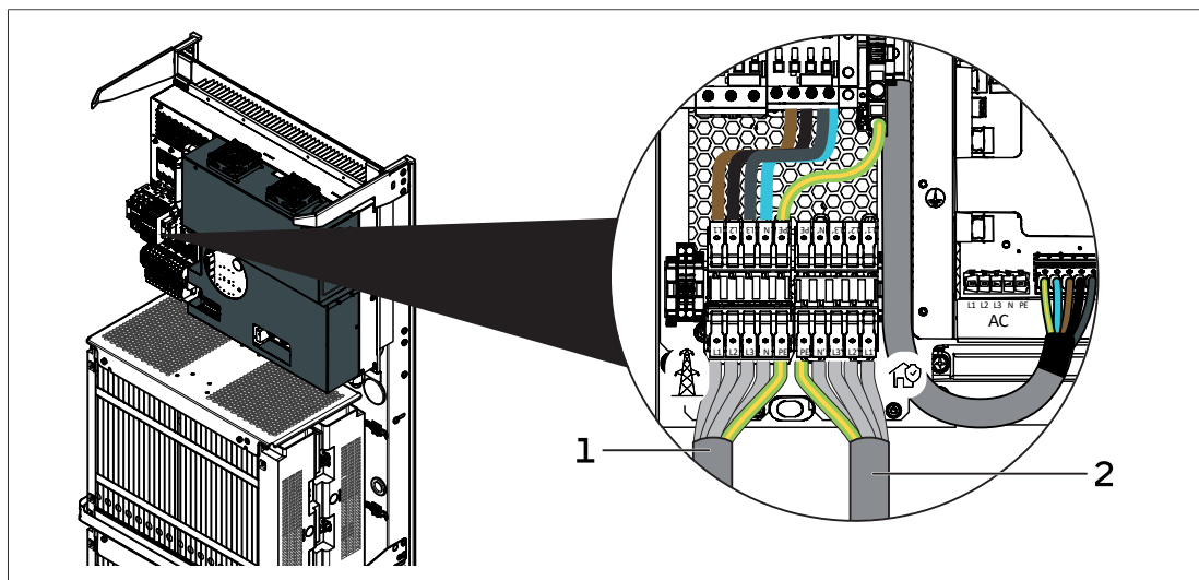
Fig. 18: Aperçu - Raccordement de la fonction électrique de secours au module de puissance
