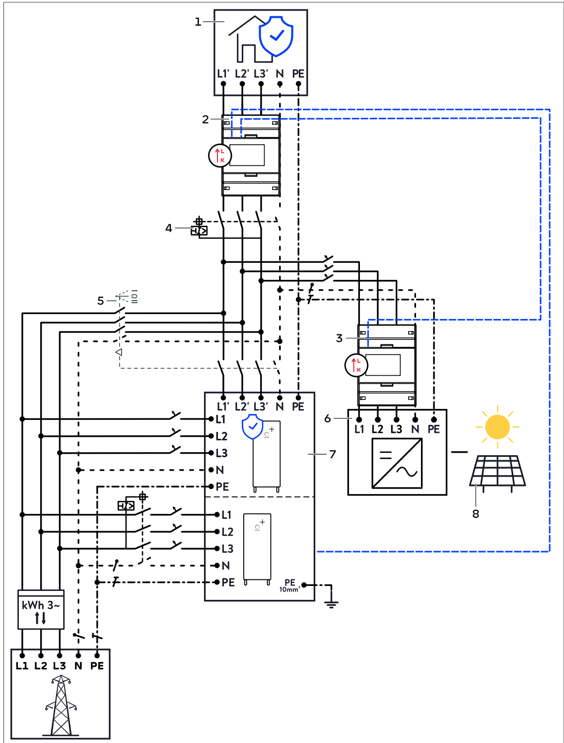
Fig. 24: Schéma de connexion général - sonnenBatterie 10 performance+ avec fonction électrique de secours - Variante de raccordement 1 avec îlot CA
