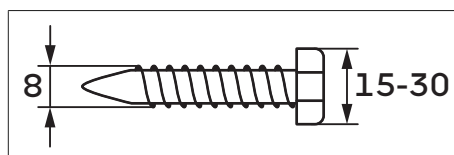
Fig. 5: Paramètres des vis à utiliser (illustration pas à l'échelle - toutes les indications sont en millimètres)
